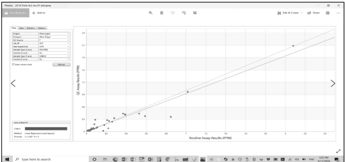
Figure 12-23: Field Duplicate Au analysis – ALS 2018
