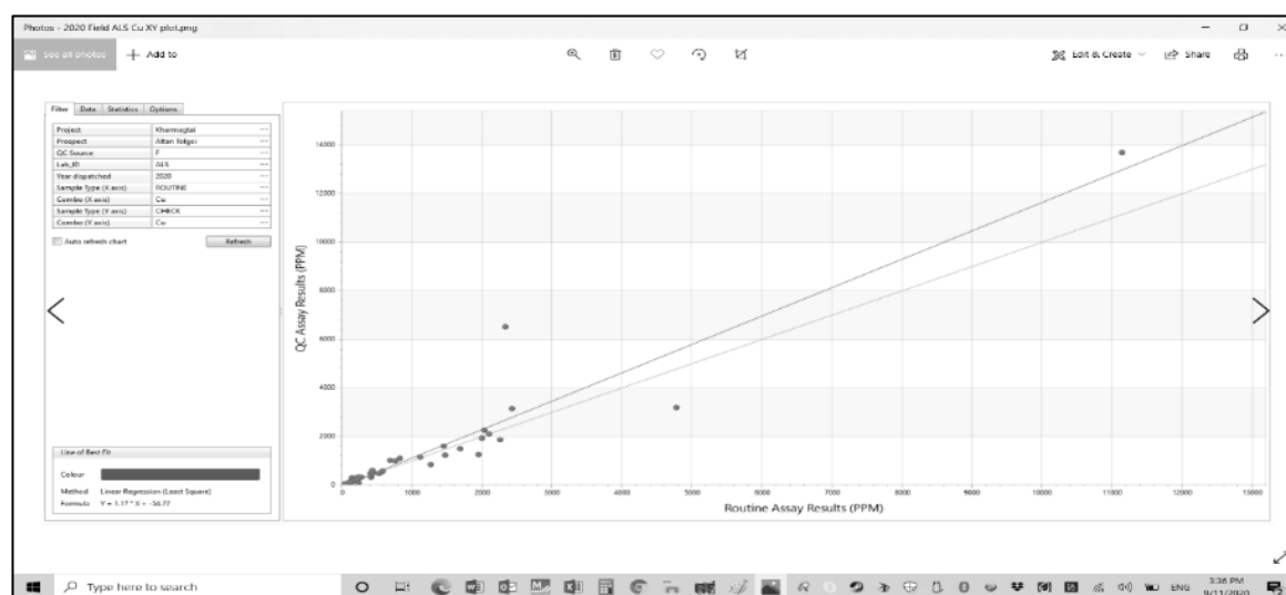
Figure 12-25: Field Duplicate Cu analysis – ALS 2020
